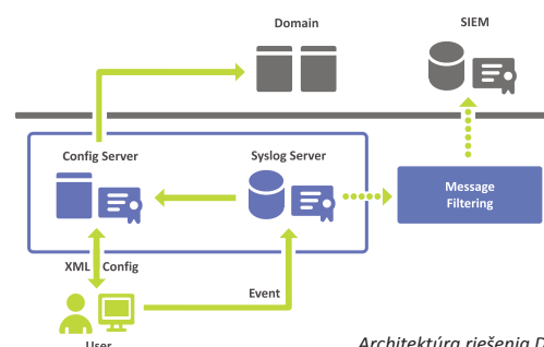
Architektúra riešenia DocTag
